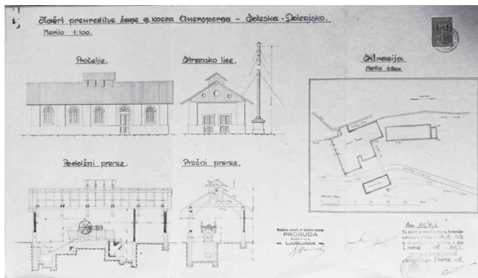
Načrt preureditve žage iz leta 1928
